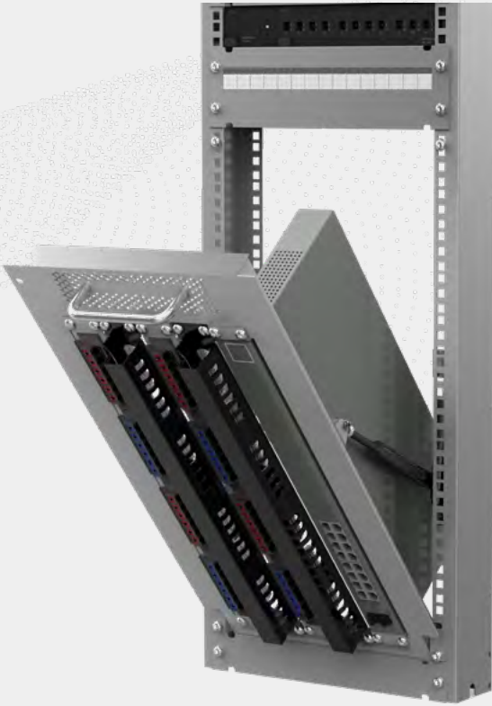
弱电模组液压门
